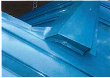
トマ-棟板金取り合い部
